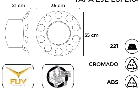
REF: 5002E TAPA EJE ESFERA
