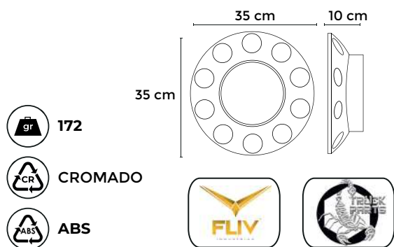
REF: 5001R TAPA RIN CILÍNDRICO
