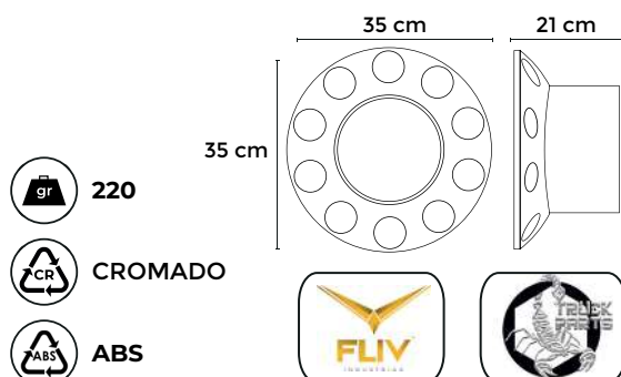
REF: 5001E TAPA EJE CILÍNDRICO
